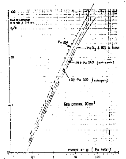
FIG.2 ETALONNAGE EN PLUTONIUM
