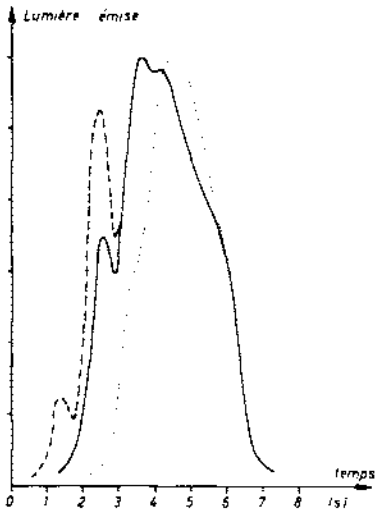
Fig. 1 Courbes de thermoluminescence ---- lecture 1 mn après irradiation ——— " 1 jour " " ..... " 1 mois " "
