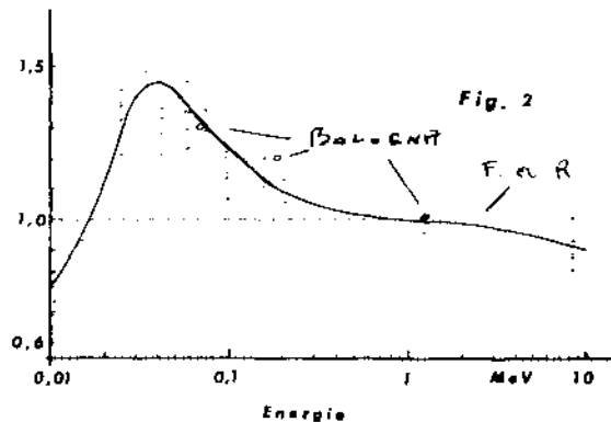
REPONSE DU FILM EN FONCTION DE L'ENERGIE
