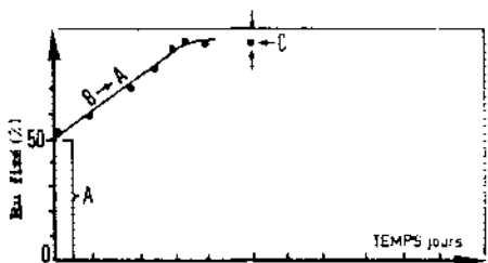
Fig. 3 Fixation (%) des complexes nitro sur TiO_2 (50 mg/litre)
