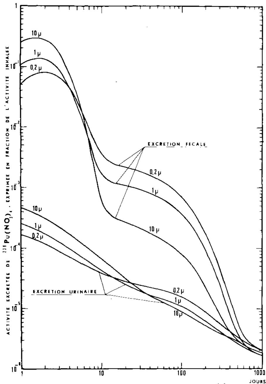
FIG. II VARIATIONS DES EXCRETIONS URINAIRE ET FECALE DE ^{239}\text{Pu}(\text{NO}_3)_4 EN FONCTION DU TEMPS APRES UNE INHALATION UNIQUE POUR 3 GRANULOMETRIES DES PARTICULES INHALEES : 0,2, 1, 10 \mu\text{m}
