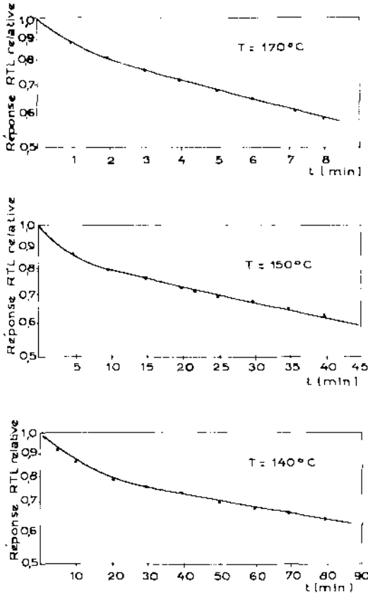
FIG 3 COURBES DE DECROISSANCE THERMIQUE
