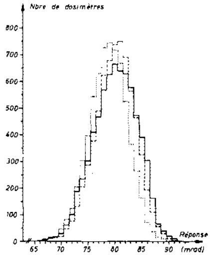
Fig. 2 Répartition de la réponse des dosimètres à 80 mrad ——— calibration originale ---- " après 1 an ..... " après 2 ans
