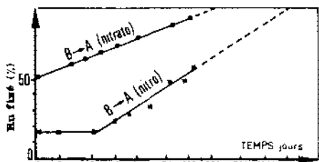
Fig. a Fixation des complexes nitro (—●—) et nitrate (—○—) par un même sédiment (2 grammes sédiment/200 cm 3 eau de mer).
