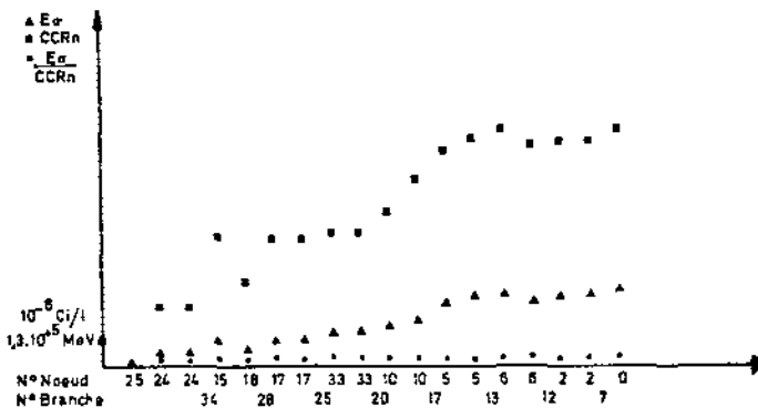
FIGURE 3 : Evolution comparées de la concentration de Radon et de l'énergie totale le long d'un chemin.
