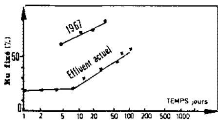
Fig. b Fixation (%) du ruthénium d'un effluent 1967 et d'un effluent actuel sur un même sédiment fixe.
