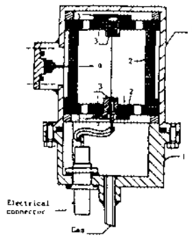
Figure 2 : Le compteur Merlin Gérin. Le volume sensible est un orthocylindre de 32,5 mm de diamètre. 1 : aluminium, 2 : plastique équivalent au tissu, 3 : isolant.
