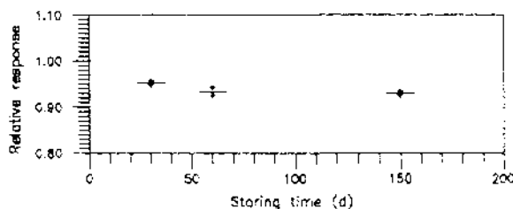
Fig. 2: Thermal fading
