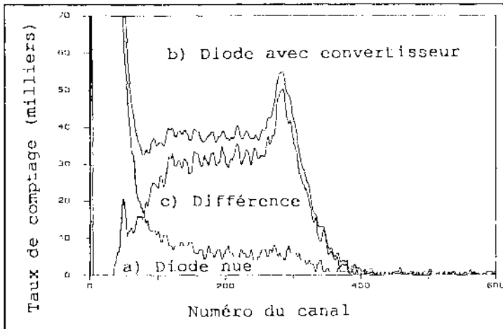
Figure 2: Réponse différentielle du système de détection, source Am-Be.
