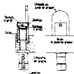
Présentation d'une broche montée sur un guide de groupe
