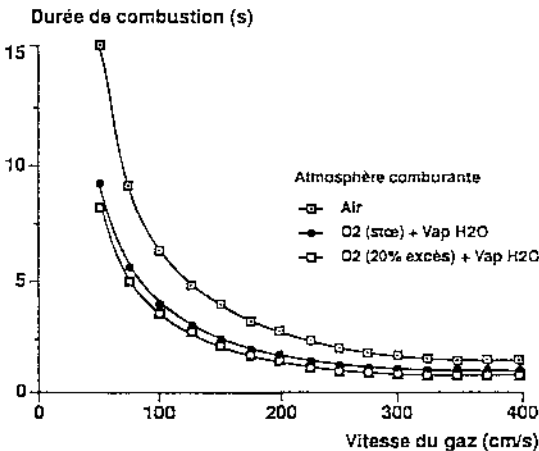
Comparaison de la cinétique de combustion d'un grain de graphite de 200 µm pour différentes compositions d'atmosphères comburantes
