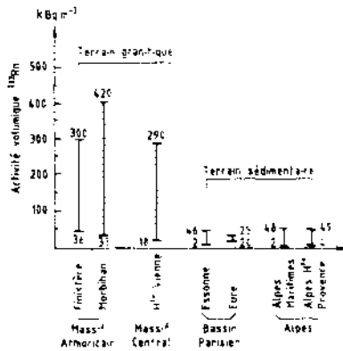
Figure 1- Activité volumique du ^{222}\text{Rn} dans les sols de différents départements français.
