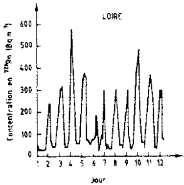
Figure 3 - Activité volumique du ^{222}\text{Rn} dans l'air extérieur à Saint-Priest-la-Prugne (département de la Loire): a) enregistrement en continu au mois de juillet 1983 b) valeurs moyennes pendant différentes périodes d'observation, d'après une mesure en continu en 1983, 1984 et 1985.
