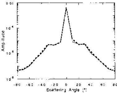
Fig. 3. BTDF of ssntd P7.
